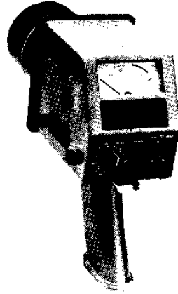
FIG. 7. Cámara de ionización (tipo Babyline).
